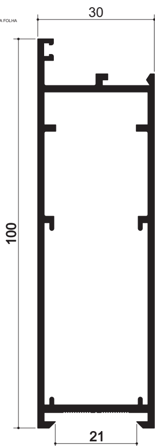
P30-082 Folha 1,086 Kg/m
