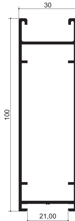
P30-377 Altura da Folha 1,081 Kg/m
