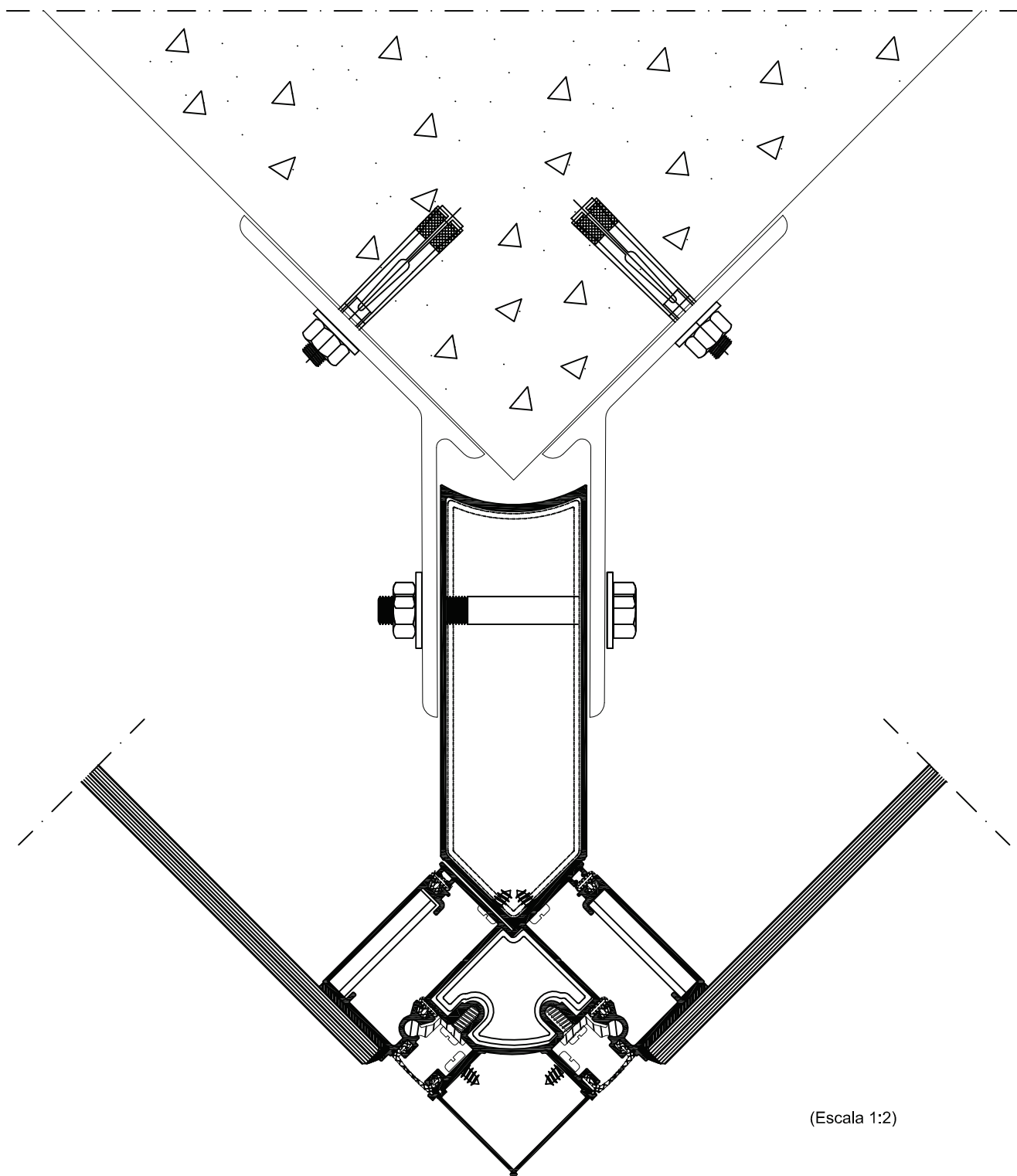
Corte 04 Lado Externo
