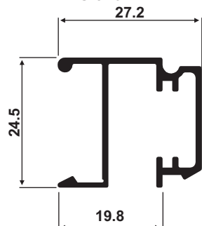
PFS-170 0,365 Kg/m
