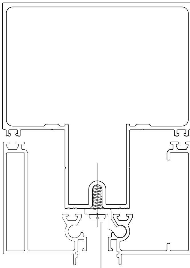
Parafuso M5 X 12 mm
