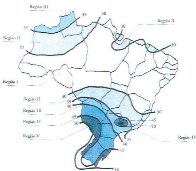
Gráfico das isoplethas da velocidade básica do vento: " v_0 " em m/s no Brasil
