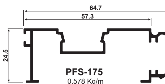
ARREMATE PISO/FORRO PARA CONTATO VIDRO
