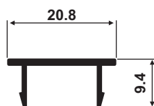
PFS-172 0,133 Kg/m
